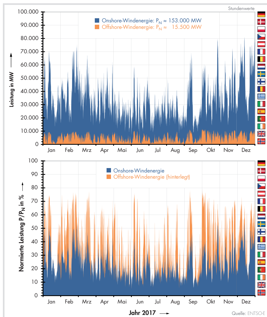
Bild 8. Summenzeitreihen der stündlichen Leistungsabgabe aus Onshore-Windenergie (blau) und Offshore-Windenergie (orange) in 18 europäischen Ländern im Jahr 2017 und normierte Summenzeitreihen unter der Annahme einer unterjährig linear wachsenden Nennleistung von Onshore-Windenergie (blau) und Offshore-Windenergie (orange, hinterlegt).
