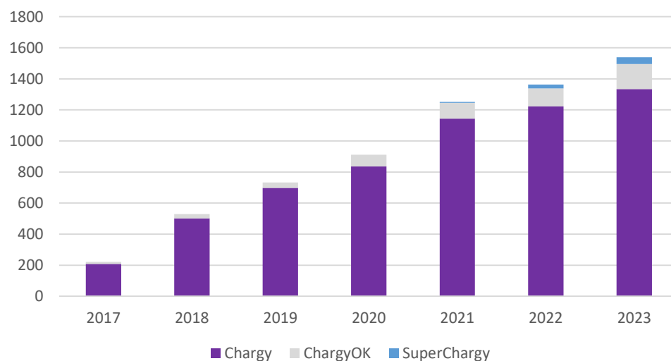
Evolution de points de charge Chargy et ChargyOK
